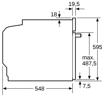
PROIEZIONE LATERALE
