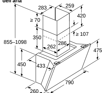
Apparecchio in modalità di estrazione dell'aria
