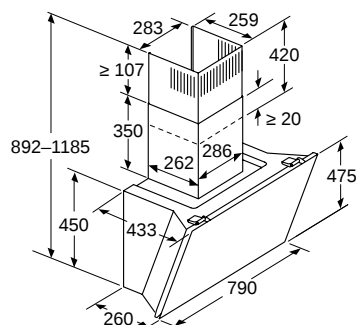
Apparecchio in modalità di ricircolo d'aria
