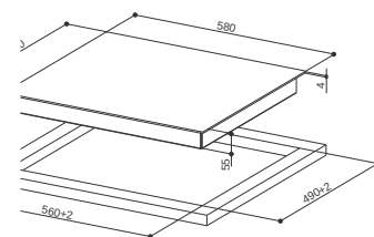
INSTALLAZIONE STANDARD
