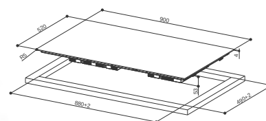
INSTALLAZIONE STANDARD
