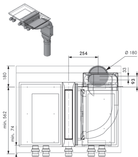
PKA3 con silenziatore piatto USDF e riduttore diritto EFRG (isola)
