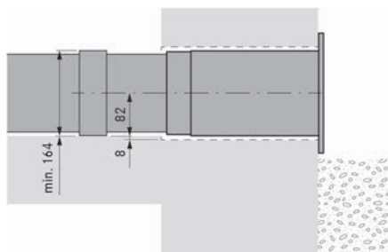
Conduzione canale sul rivestimento del pavimento
